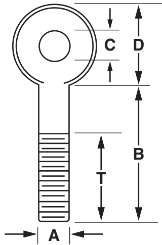
Rod End
